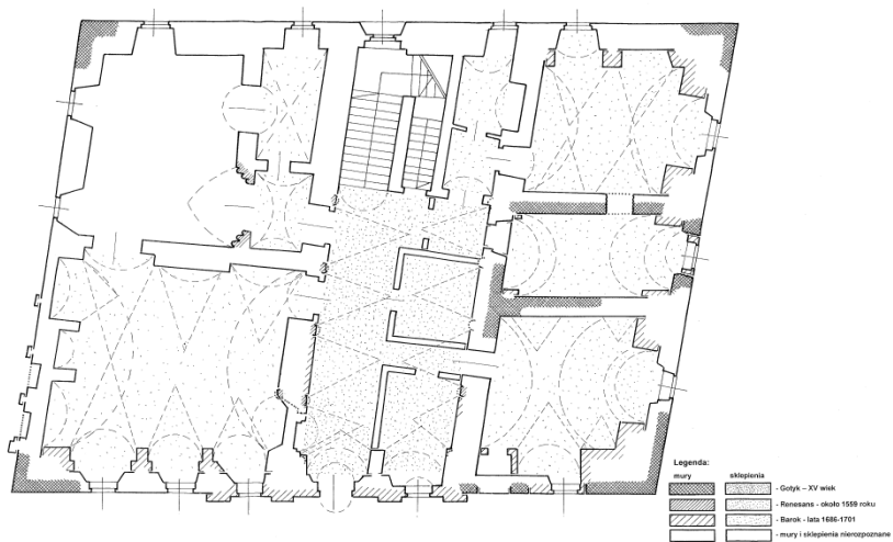
Ryc. 4. Grobniki, Komenda, rzut parteru z chronologicznym rozwarstwieniem murów.
