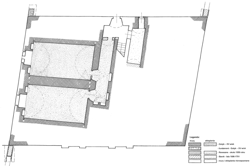
Ryc. 3. Grobniki, Komenda, rzut piwnic z chronologicznym rozwarstwieniem murów.
